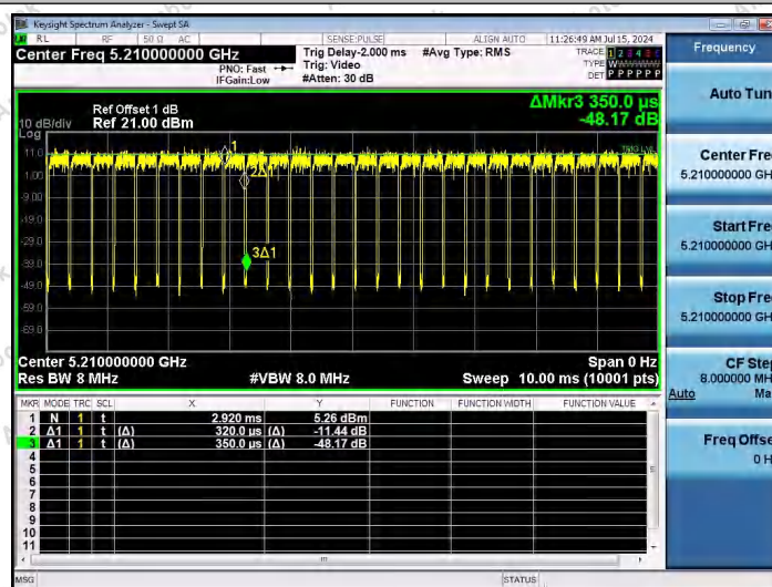
NTNV-11AC80SISO-Ant1-5210
