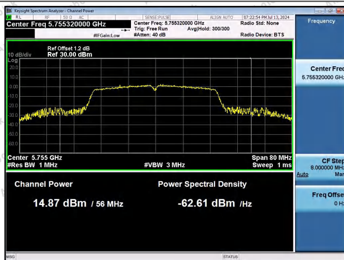
11N40SISO-Ant1-5755-PASS
