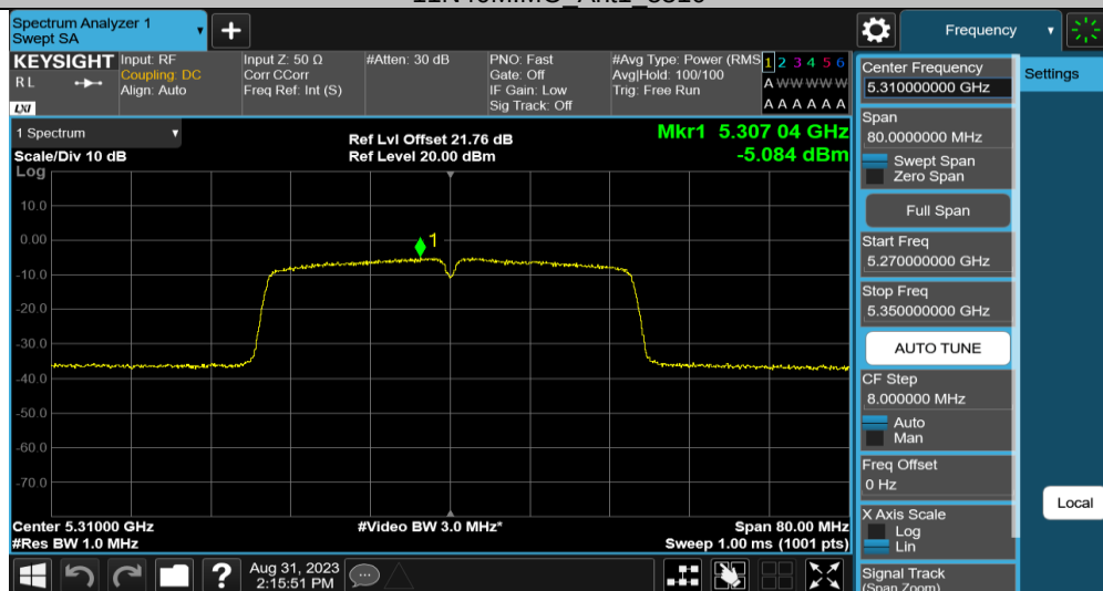
11N40MIMO Ant2 5310
