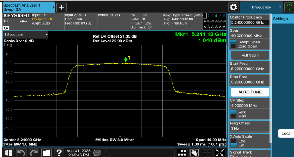
11AC20MIMO_Ant2_5240
