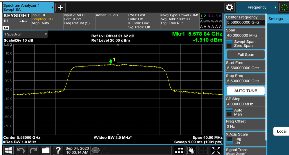
11AC20MIMO_Ant2_5580
