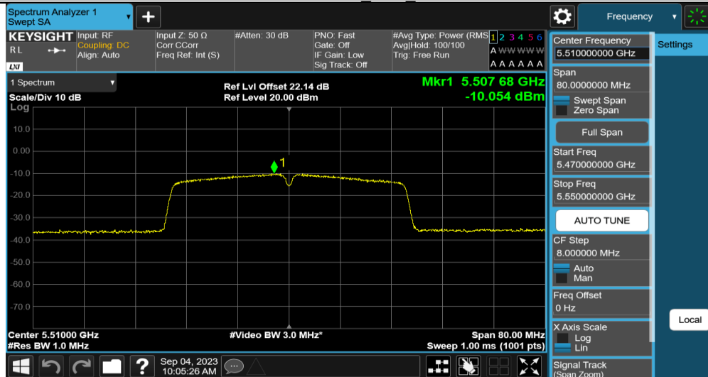
11N40MIMO Ant2 5510
