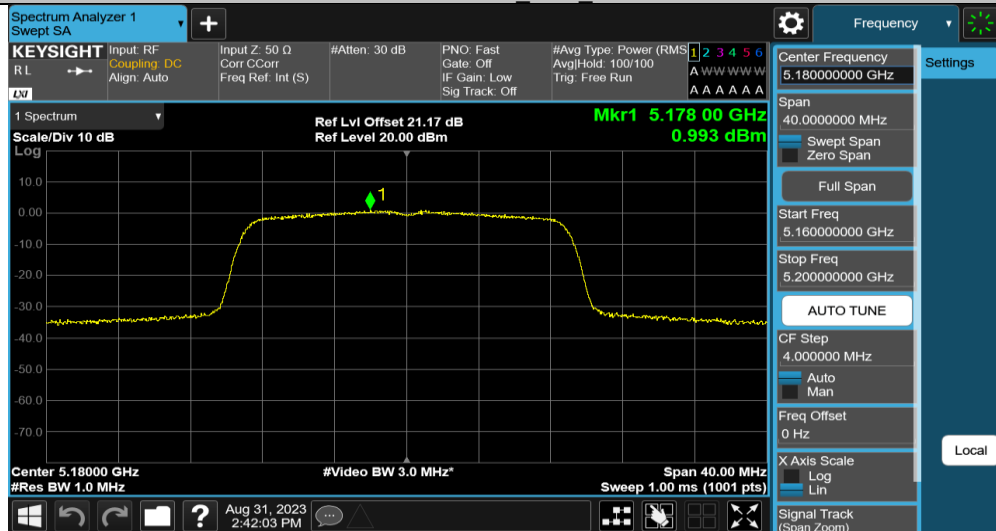
11AC20MIMO_Ant2_5180
