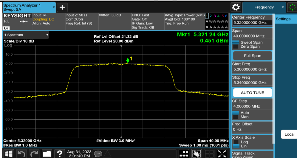
11AC20MIMO_Ant2_5320
