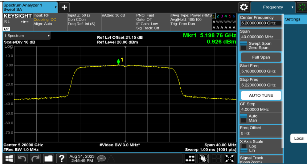
11AC20MIMO_Ant2_5200
