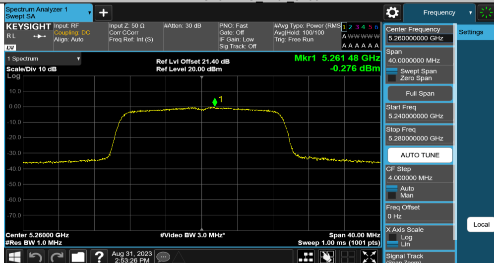
11AC20MIMO_Ant2_5260
