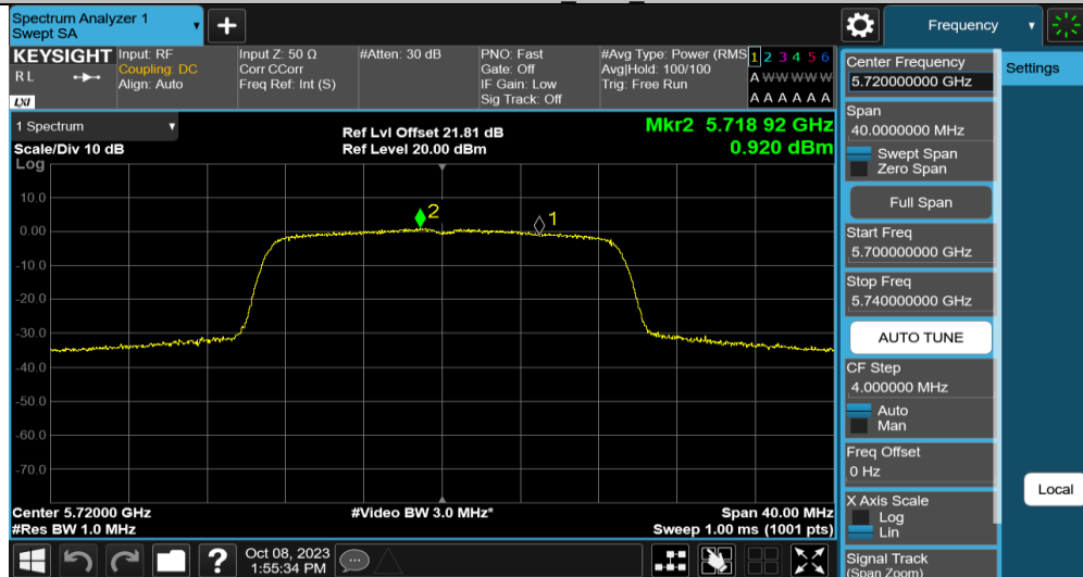
11AC20MIMO_Ant2_5720
