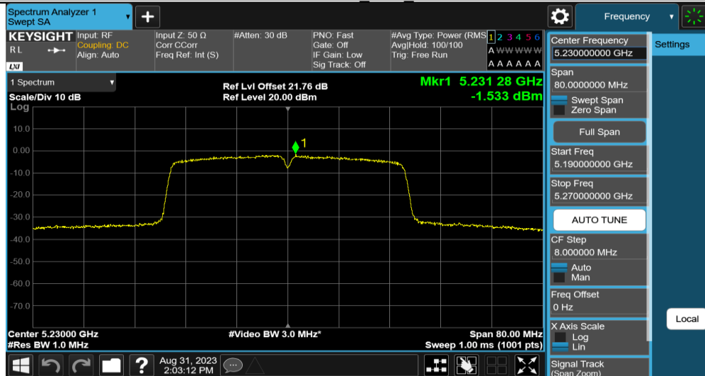
11N40MIMO Ant2 5230
