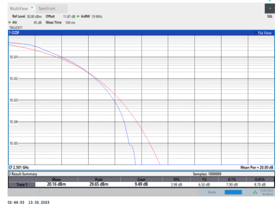
Band41-10MHz-QPSK-39700-50RB#0
