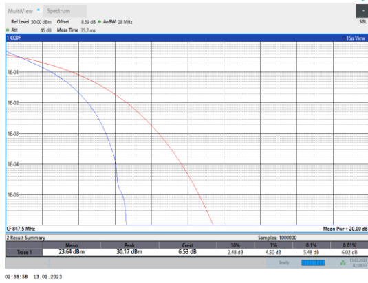
Band5-3MHz-QPSK-20635-15RB#0
