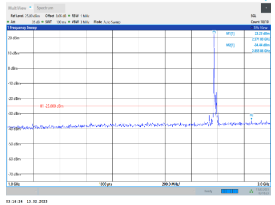
Band38-20MHz-QPSK-37850-1RB#0-Range2:1000~3000MHz
