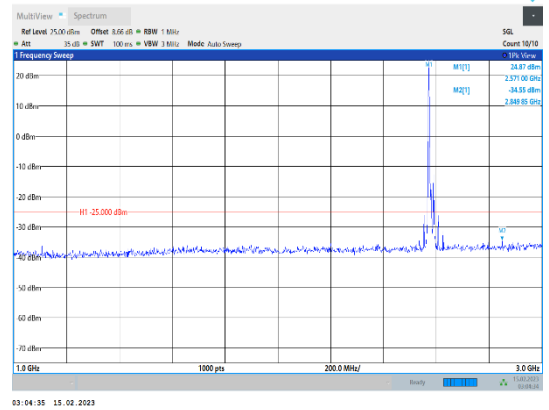
Band38-20MHz-64QAM-37850-1RB#0-Range2:1000~3000MHz
