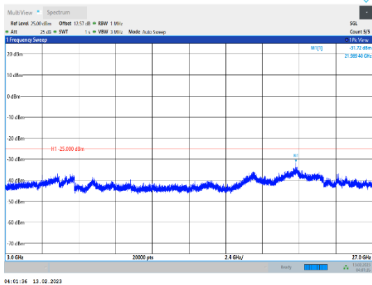
Band41-5MHz-QPSK-39675-1RB#0-Range3:3000~27000MHz
