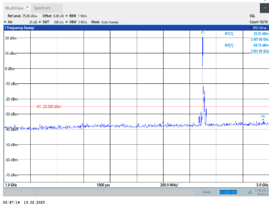
Band41-15MHz-QPSK-39725-1RB#0-Range2:1000~3000MHz
