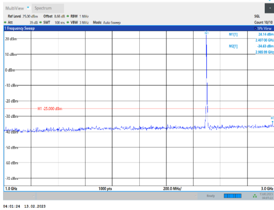
Band41-5MHz-QPSK-39675-1RB#0-Range2:1000~3000MHz
