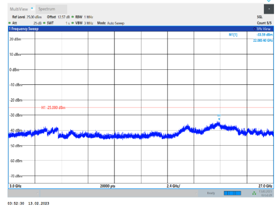
Band41-10MHz-QPSK-41540-1RB#0-Range3:3000~27000MHz
