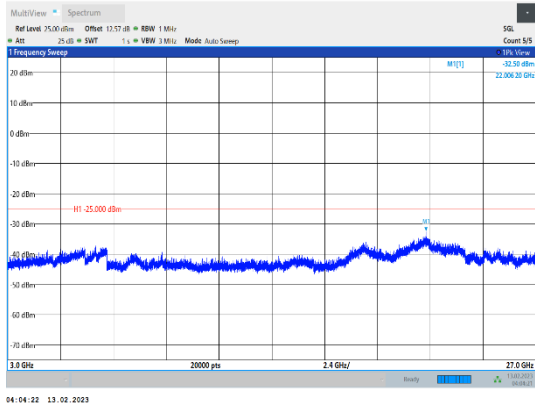
Band41-5MHz-QPSK-41565-1RB#0-Range3:3000~27000MHz
