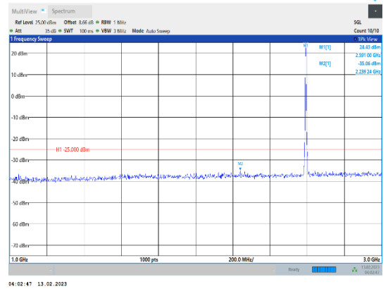
Band41-5MHz-QPSK-40620-1RB#0-Range2:1000~3000MHz
