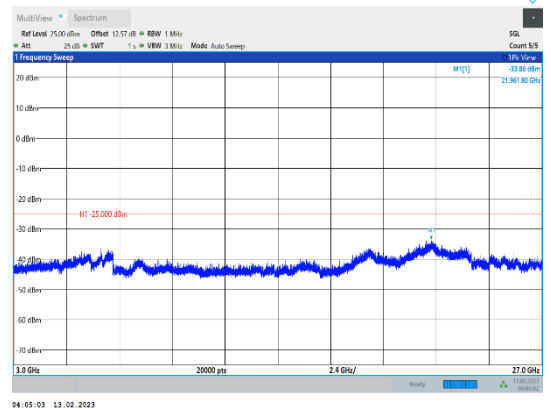
Band41-5MHz-16QAM-41565-1RB#0-Range3:3000~27000MHz
