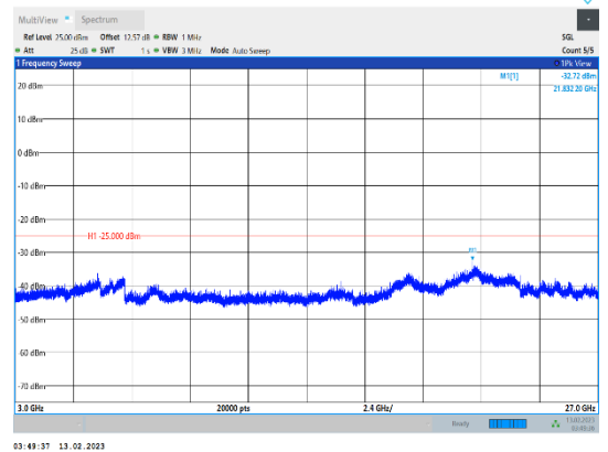
Band41-10MHz-QPSK-39700-1RB#0-Range3:3000~27000MHz
