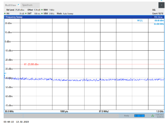
Band41-10MHz-QPSK-39700-1RB#0-Range1:30~1000MHz
