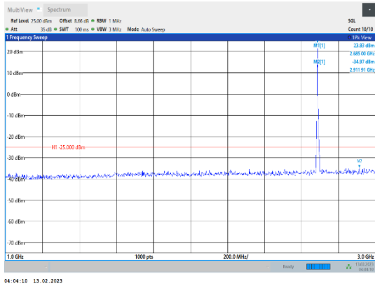
Band41-5MHz-QPSK-41565-1RB#0-Range2:1000~3000MHz
