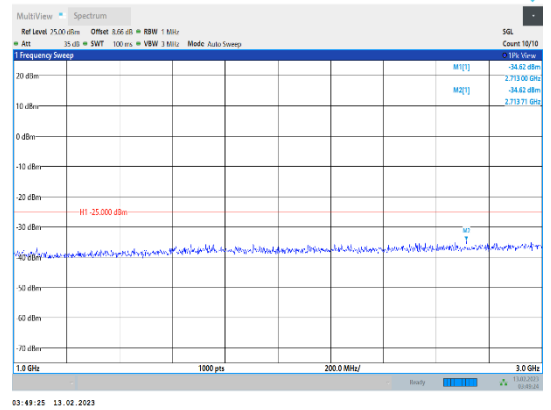
Band41-10MHz-QPSK-39700-1RB#0-Range2:1000~3000MHz
