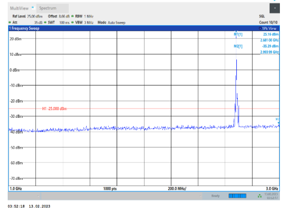
Band41-10MHz-QPSK-41540-1RB#0-Range2:1000~3000MHz
