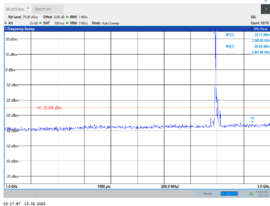
Band38-20MHz-QPSK-38000-1RB#0-Range2:1000~3000MHz
