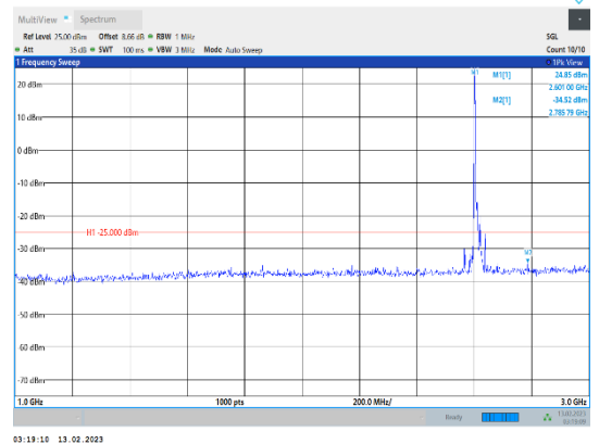
Band38-20MHz-QPSK-38150-1RB#0-Range2:1000~3000MHz
