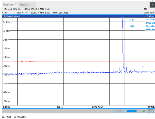
Band38-20MHz-16QAM-37850-1RB#0-Range2:1000~3000MHz
