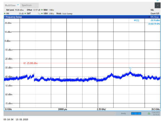
Band38-20MHz-QPSK-37850-1RB#0-Range3:3000~26500MHz
