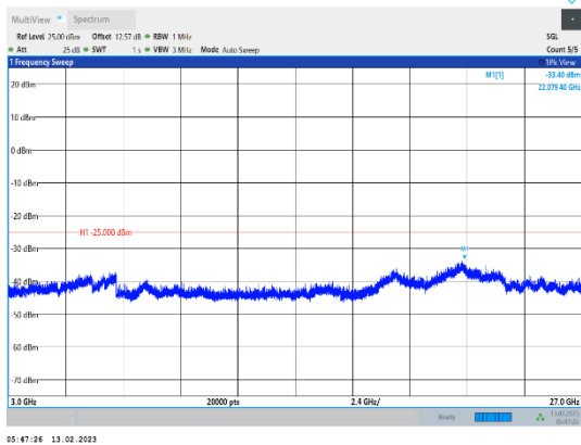
Band41-15MHz-QPSK-39725-1RB#0-Range3:3000~27000MHz
