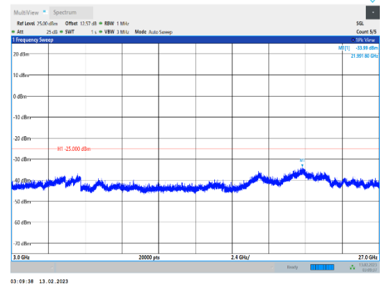
Band41-20MHz-QPSK-41490-1RB#0-Range3:3000~27000MHz
