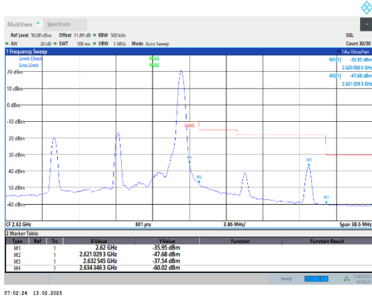
Band38-15MHz-QPSK-38175-1RB#74
