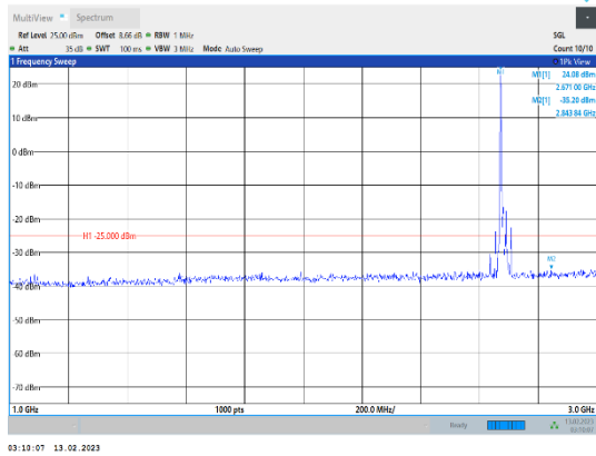
Band41-20MHz-16QAM-41490-1RB#0-Range2:1000~3000MHz
