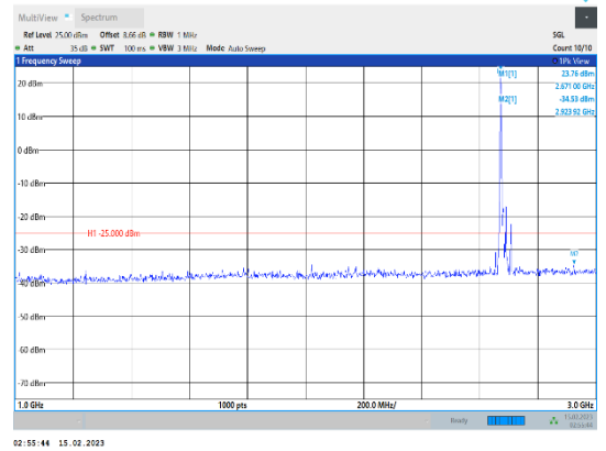
Band41-20MHz-64QAM-41490-1RB#0-Range2:1000~3000MHz
