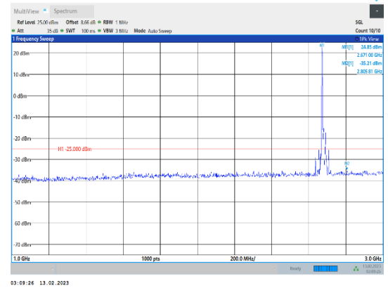
Band41-20MHz-QPSK-41490-1RB#0-Range2:1000~3000MHz
