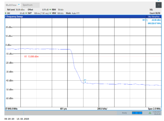
Band5-3MHz-QPSK-20635-15RB#0
