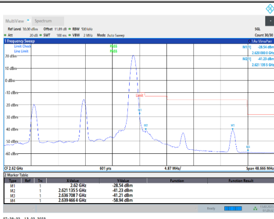
Band38-20MHz-QPSK-38150-1RB#99
