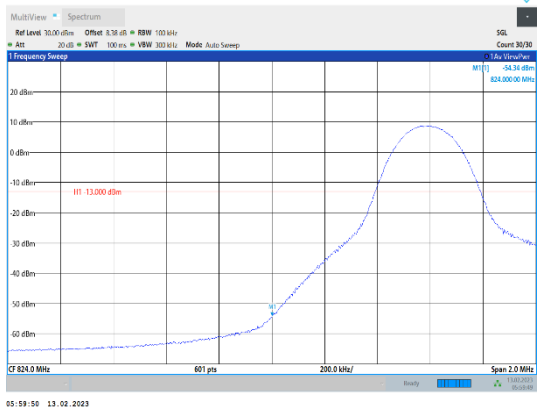
Band5-10MHz-QPSK-20450-1RB#0
