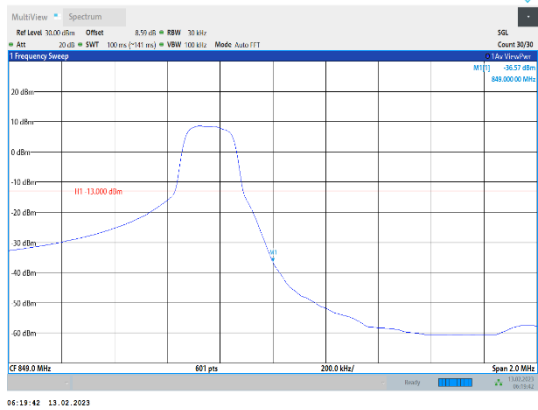
Band5-3MHz-QPSK-20635-1RB#14
