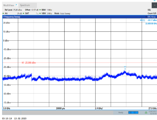
Band41-20MHz-16QAM-41490-1RB#0-Range3:3000~27000MHz
