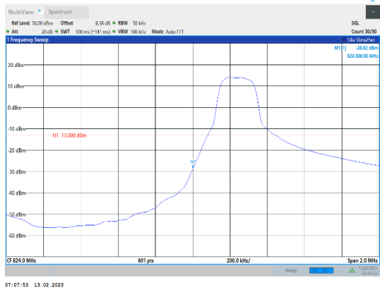
Band5-3MHz-QPSK-20415-1RB#0
