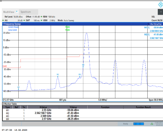
Band38-20MHz-QPSK-37850-1RB#0
