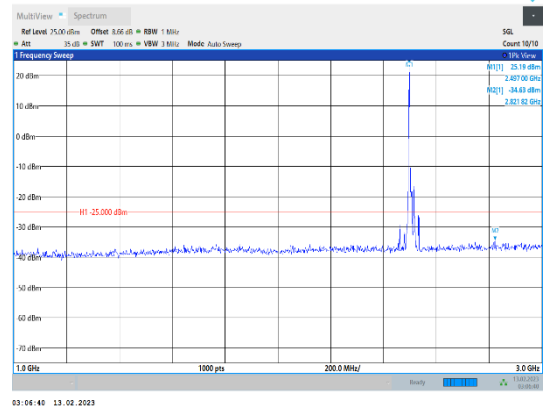
Band41-20MHz-QPSK-39750-1RB#0-Range2:1000~3000MHz
