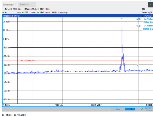
Band41-20MHz-QPSK-40620-1RB#0-Range2:1000~3000MHz
