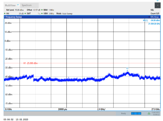
Band41-20MHz-QPSK-39750-1RB#0-Range3:3000~27000MHz
