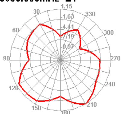
5650.000MHz E1
