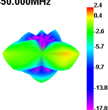
2450.000MHz
