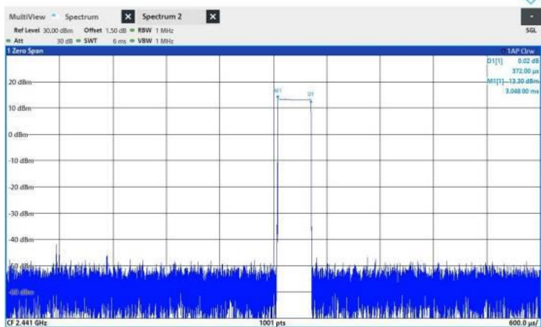
DH1_Ant1_Hop
