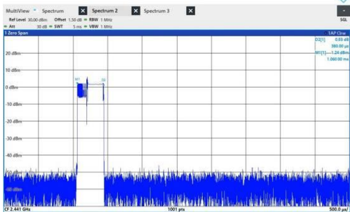
2DH1_Ant1_Hop
