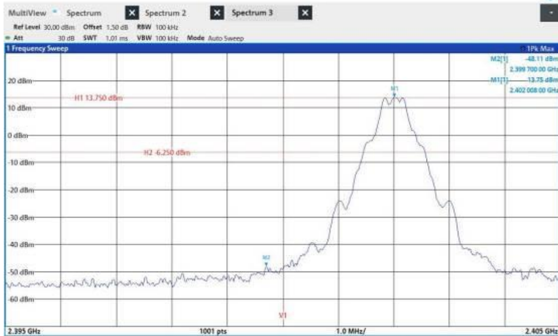
DH5_Ant1_Low_2402
