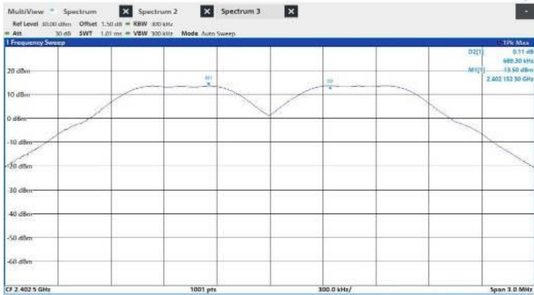
DH5_Ant1_Hop
