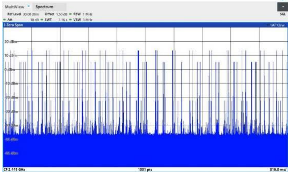
DH1_Ant1_Hop
