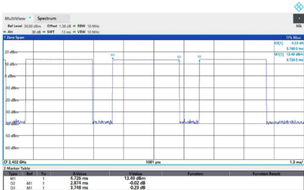
DH5_Ant1_2402
