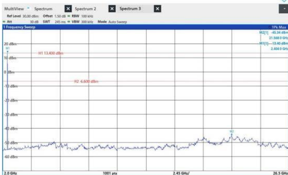
DH5_Ant1_2402_2000~26500
