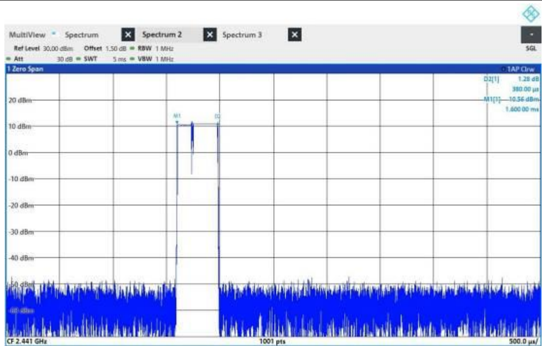
3DH1_Ant1_Hop
