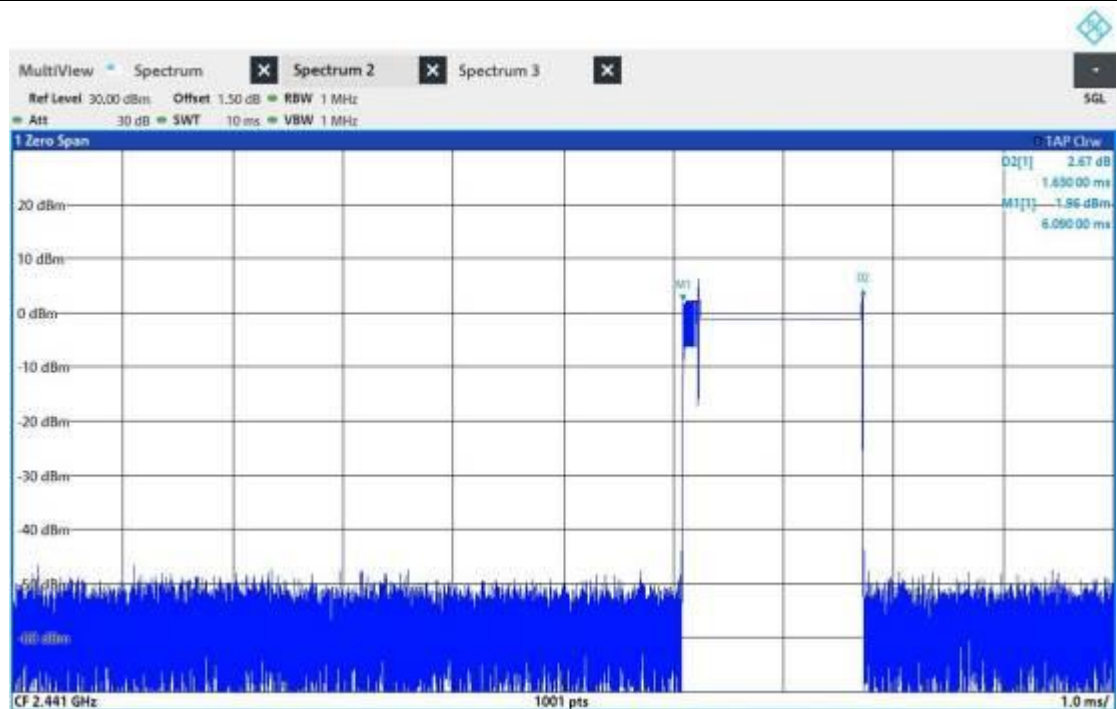
3DH3_Ant1_Hop
