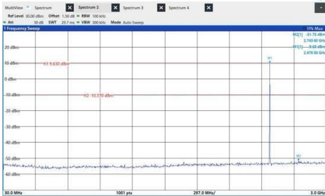
3DH5_Ant1_2480_30~3000
