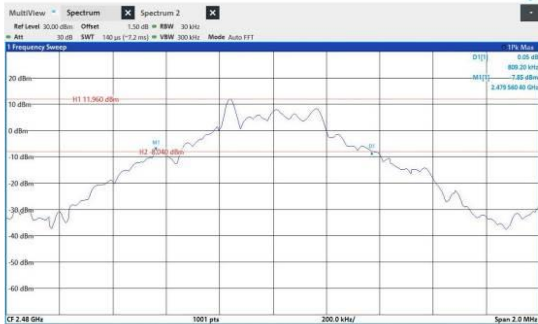
DH5_Ant1_2480
