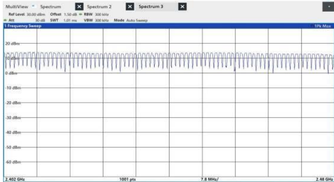
DH5_Ant1_Hop
