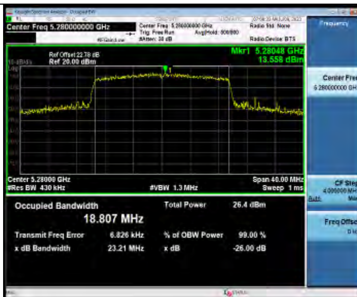
11AX20MIMO_Ant2_5280
