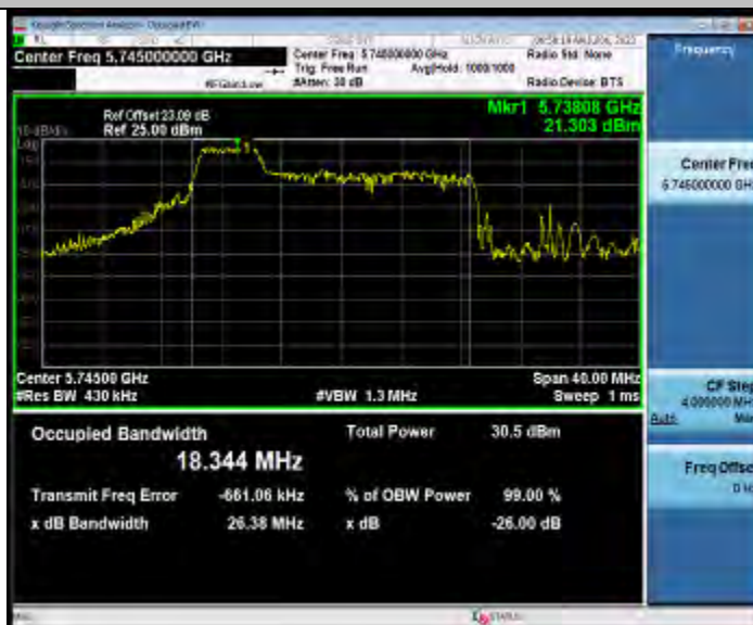
11AX20MIMO_Ant1_5745_106Tone_RU53
