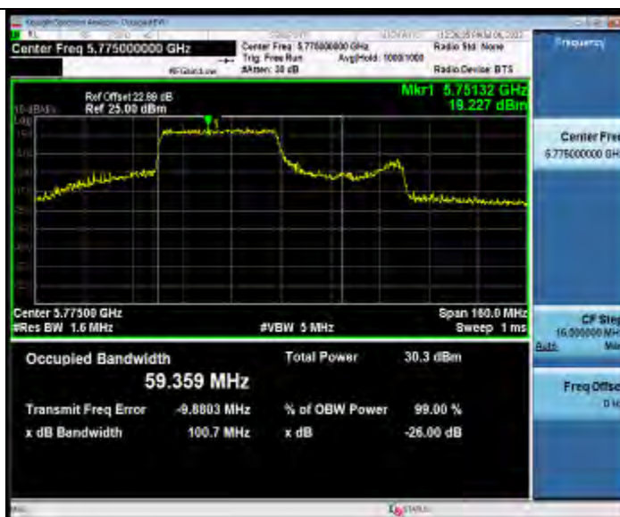
11AX80MIMO_Ant2_5775_996Tone_RU67
