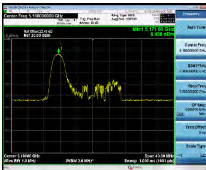
11AX20MIMO_Ant2_5180_52Tone_RU37
