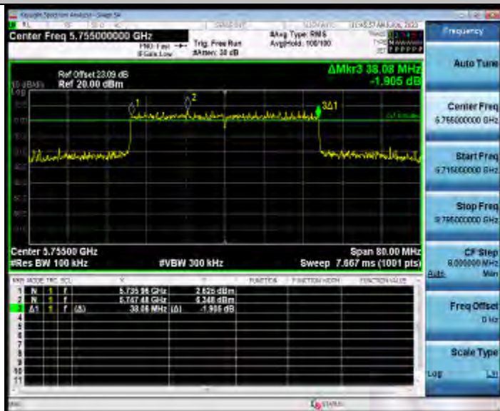
11AX40MIMO_Ant2_5755_242Tone_RU61
