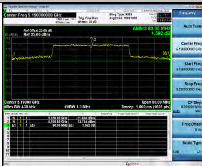
11AX40MIMO_Ant2_5190_242Tone_RU61
