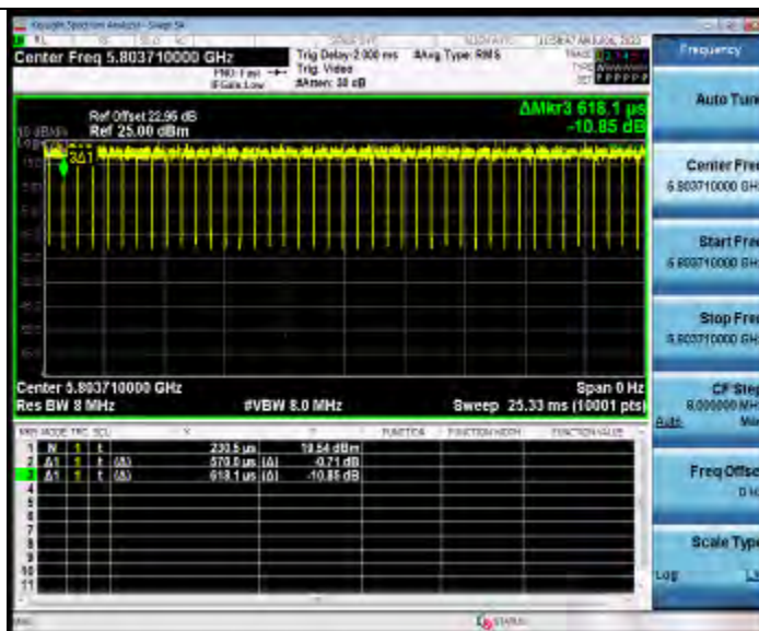
11AX40MIMO_Ant2_5795_484Tone_RU65
