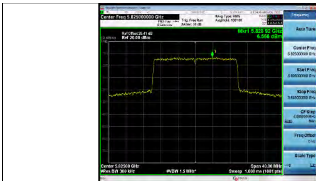
11AX20MIMO_Ant2_5825_242Tone_RU61
