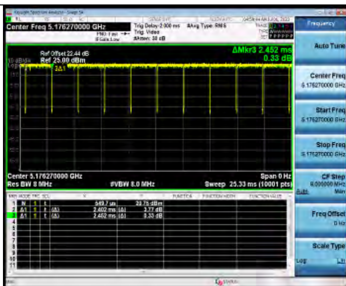
11AX20MIMO_Ant2_5180_242Tone_RU61
