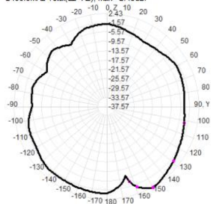
2480.0MHz Total(E2-YZ), Max= 2.43dBi
