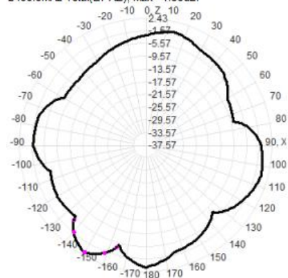
2480.0MHz Total(E1-XZ), Max= 1.36dBi
