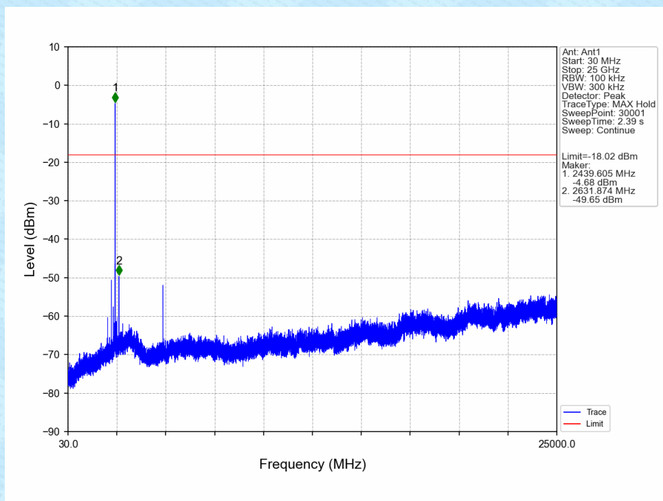
2M_MCH_2440MHz_Ant1_NTNV
