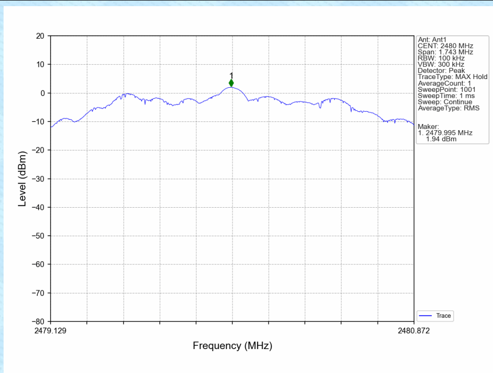
2M_HCH_2480MHz_Ant1_NTNV
