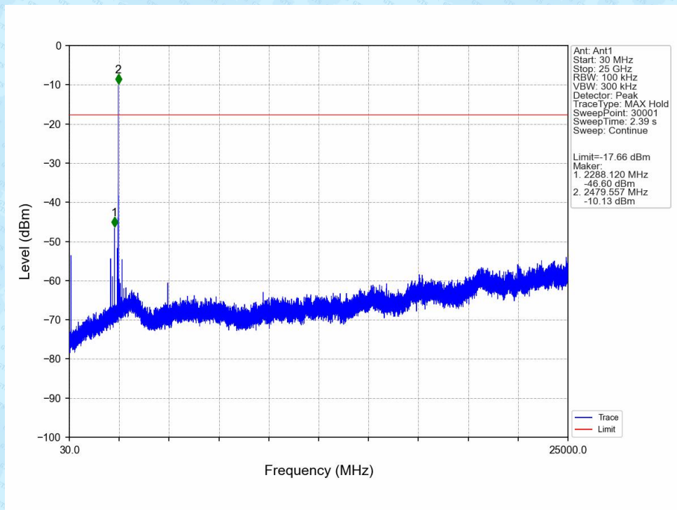
2M_HCH_2480MHz_Ant1_NTNV
