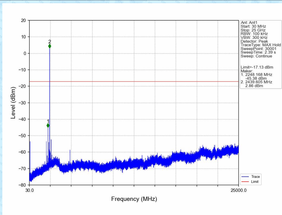
2M_MCH_2440MHz_Ant1_NTNV
