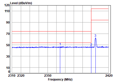
2.4G SRD_TX_CH_L_Vertical
