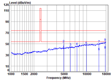
2.4G SRD_TX_CH_H_Vertical
