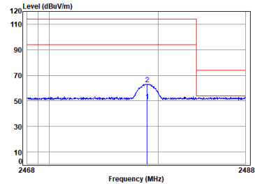
2.4G SRD_TX_CH_H_Vertical
