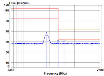
2.4G SRD_TX_CH_H_Vertical
