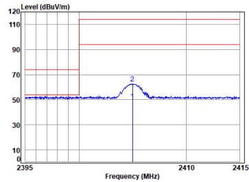
2.4G SRD_TX_CH_L_Vertical
