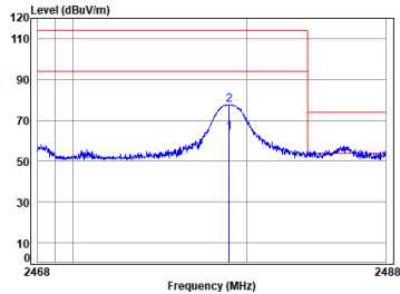
2.4G SRD_TX_CH_H_Horizontal
