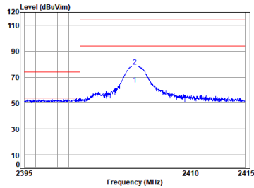
2.4G SRD_TX_CH_L_Horizontal
