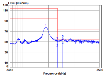
2.4G SRD_TX_CH_H_Horizontal
