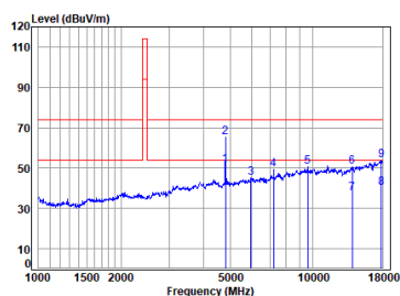
2.4G SRD_TX_CH_L_Horizontal
