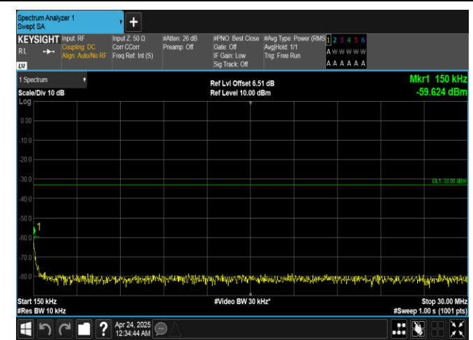
Band25-20MHz-QPSK-26365-1RB#99-0.15~30-PASS
