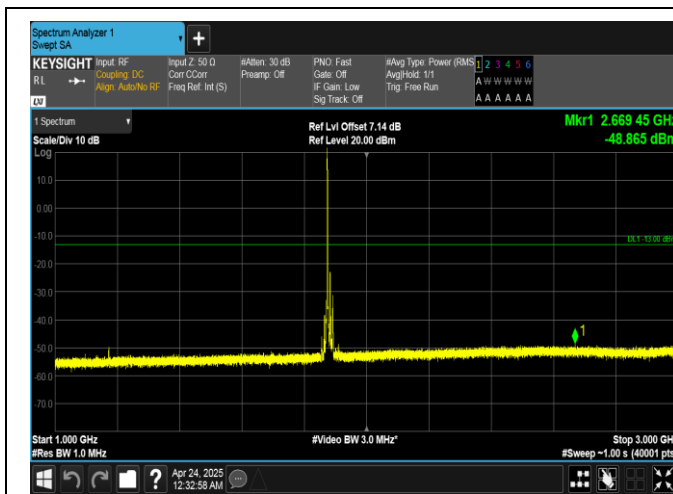
Band25-20MHz-QPSK-26365-1RB#0-1000~3000-PASS
