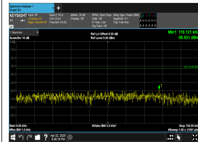
Band5-3MHz-QPSK-20635-15RB#0-0.009~0.15-PASS
