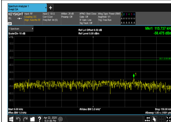
Band5-3MHz-QPSK-20635-1RB#0-0.009~0.15-PASS
