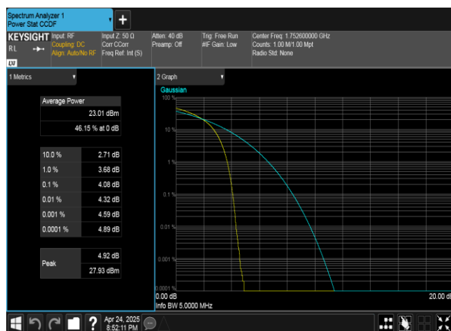
Band4-1513-5-PASS
