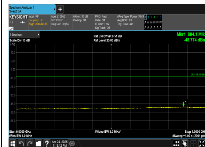
Band4-1513-30~1000MHz-PASS
