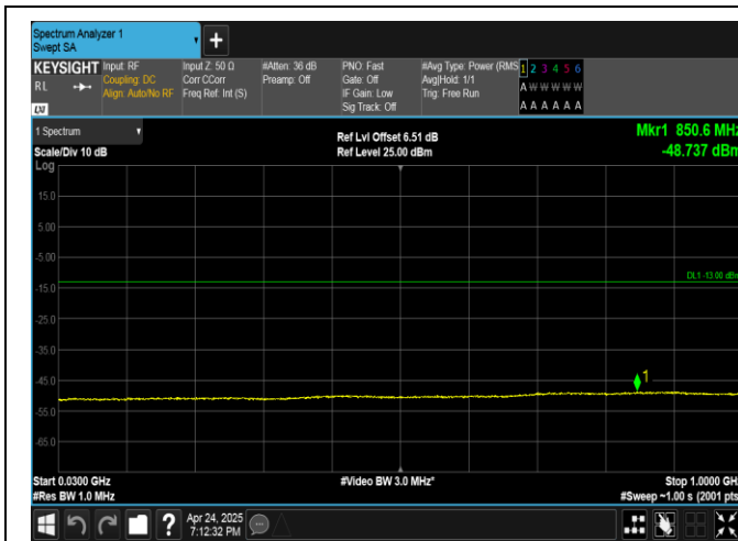
Band4-1413-30~1000MHz-PASS
