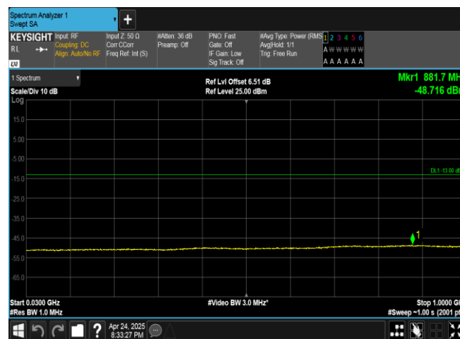
Band4-1312-3-30~1000MHz-PASS
