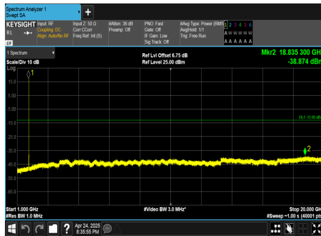
Band4-1312-4-1000~20000MHz-PASS
