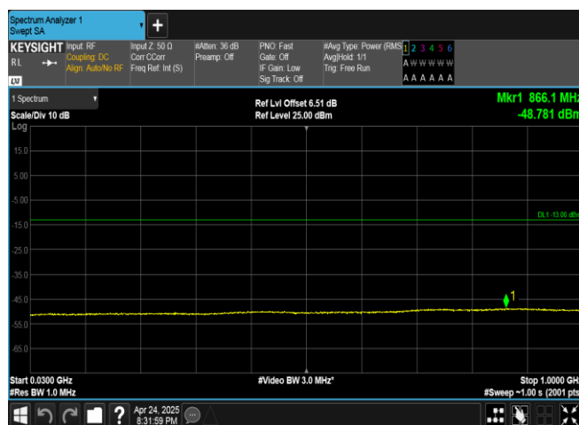
Band4-1513-2-30~1000MHz-PASS
