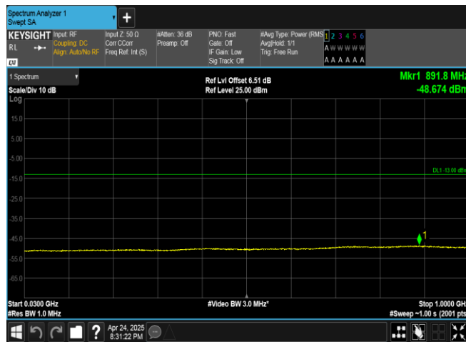
Band4-1413-2-30~1000MHz-PASS
