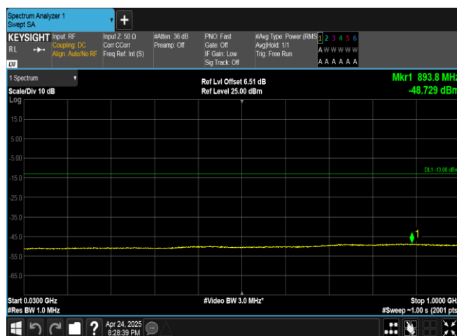
Band4-1312-1-30~1000MHz-PASS
