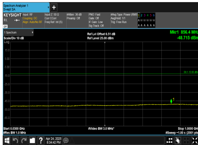
Band4-1513-3-30~1000MHz-PASS
