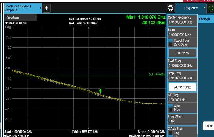
1RB (1902.5MHz)
