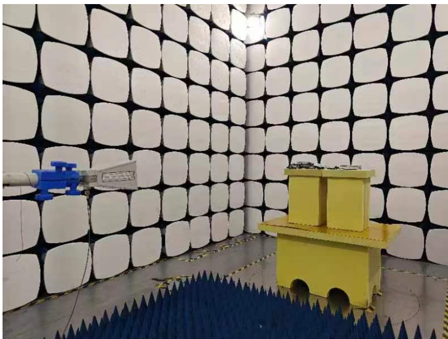
1GHz-18GHz
