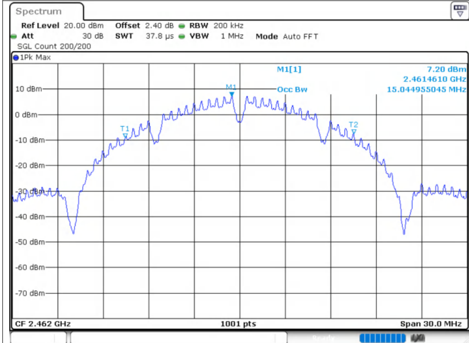
OBW NVNT b 2462MHz Ant1
