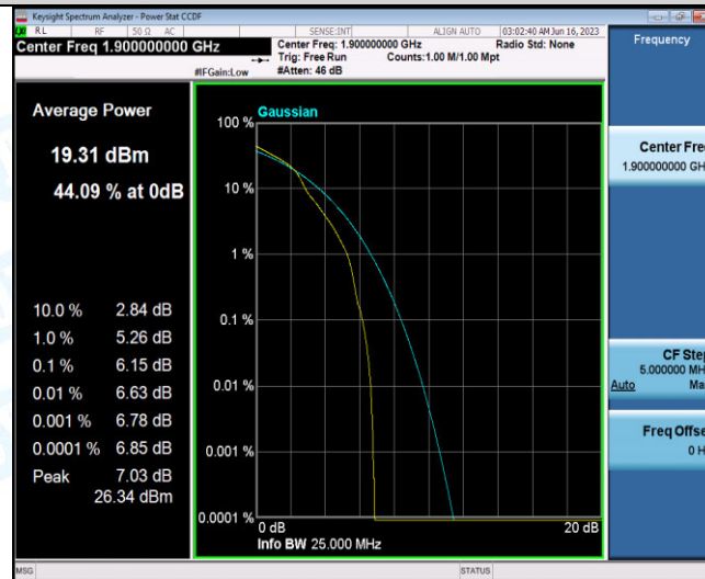
Band2-20MHz-16QAM-19100-27RB#0
