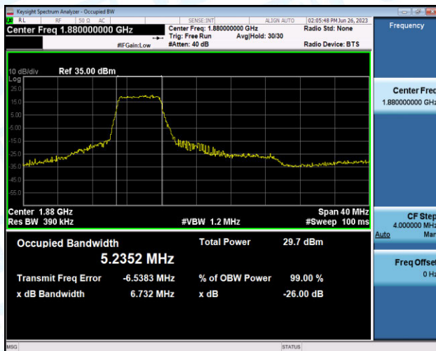
Band2-20MHz-16QAM-18900-27RB#0-PASS
