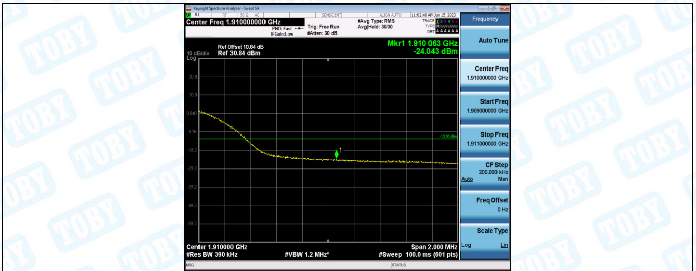
Band2-20MHz-16QAM-18700-27RB#0
