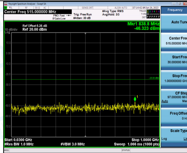
Band41-5MHz-QPSK-40065-1RB#0-Range1:30~1000MHz
