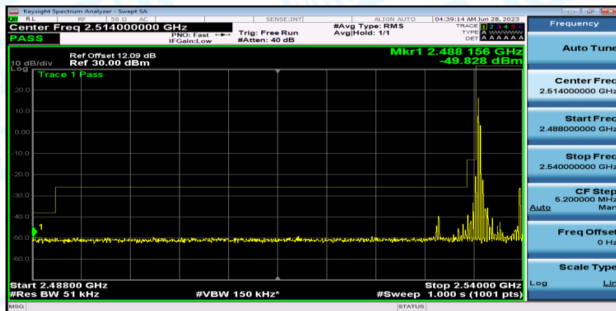
Band41_Band41_5MHz_QPSK_40065_1RB#0
