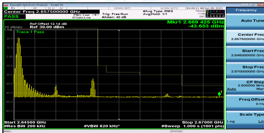
Band41_Band41_10MHz_QPSK_41190_1RB#0
