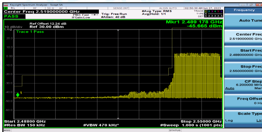
Band41_Band41_15MHz_QPSK_40115_75RB#0
