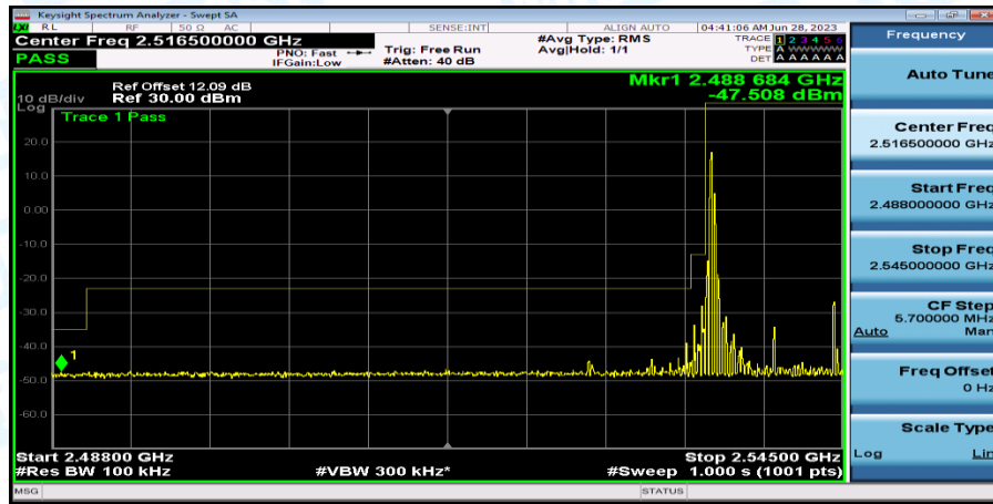
Band41_Band41_10MHz_QPSK_40090_1RB#0
