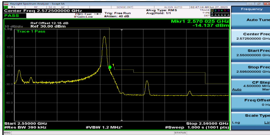
Band7_20MHz_QPSK_21350_1RB#99
