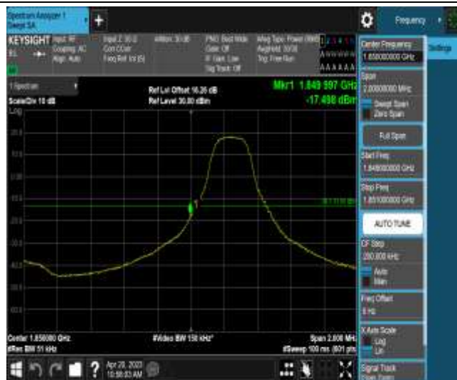
Band2-3MHz-QPSK-18615-1RB#0
