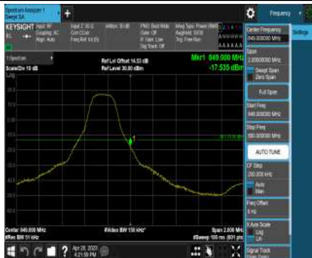
Band5-3MHz-QPSK-20635-1RB#14
