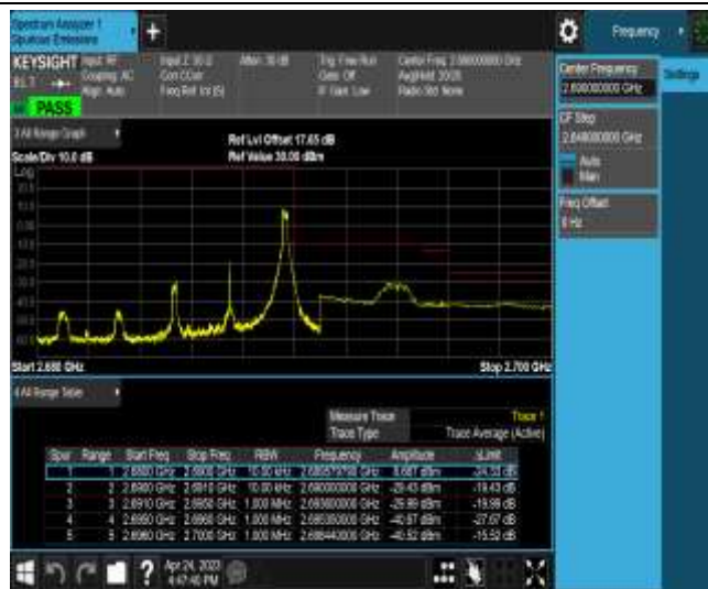
Band41-5MHz-16QAM-41565-1RB#24
