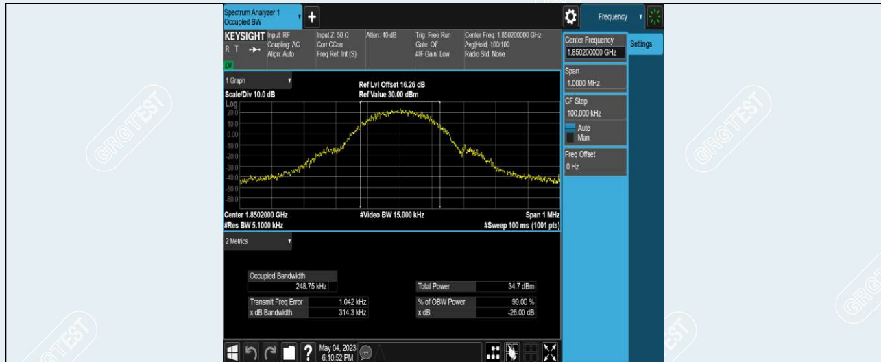
GPRS1900-512
