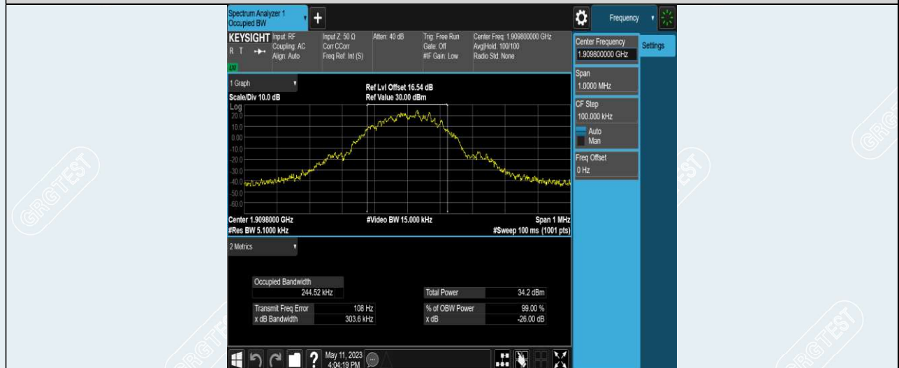
PCS1900-810
