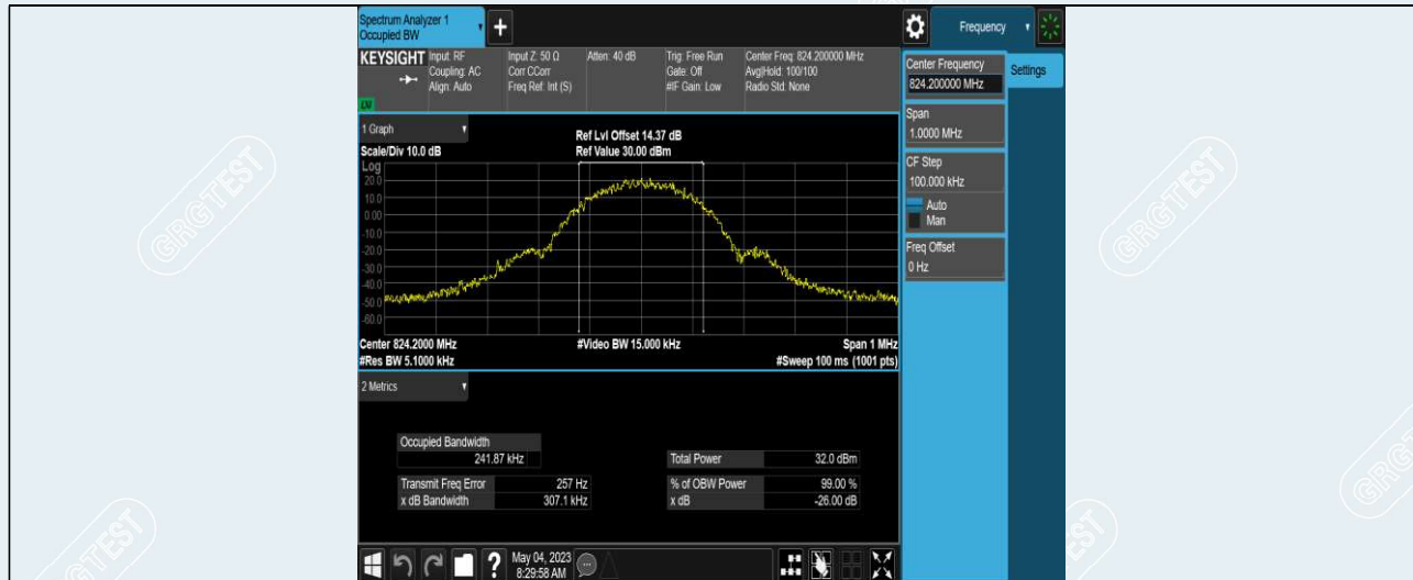
EGPRS850-128
