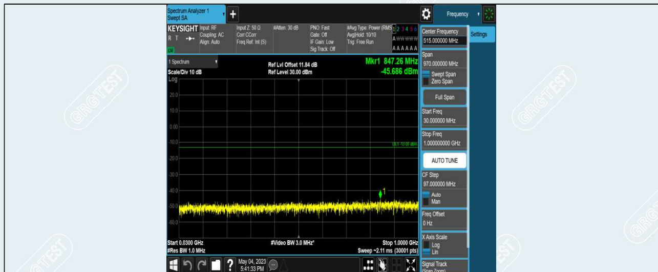
PCS1900-512-30~1000MHz
