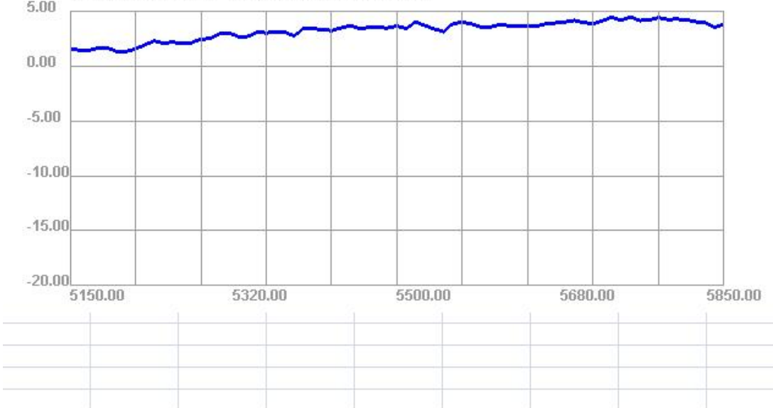
5150.00MHz - 5850.00MHz Efficiency
