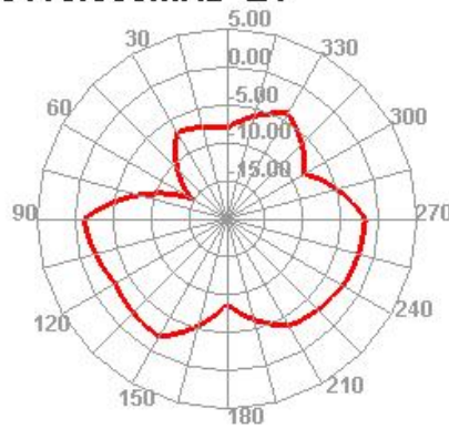
5160.000MHz E1
