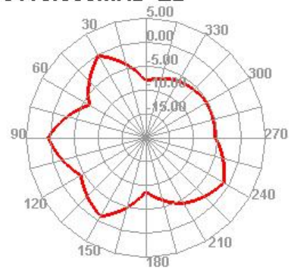
5160.000MHz E2
