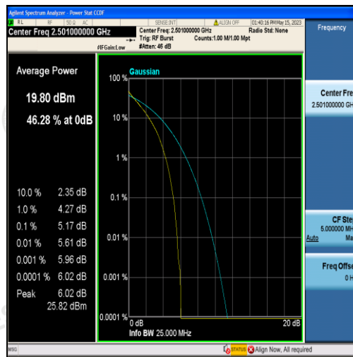
Band41-10MHz-QPSK-39700-50RB#0
