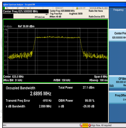
Band5-3MHz-QPSK-20415-15RB#0-2.6895
