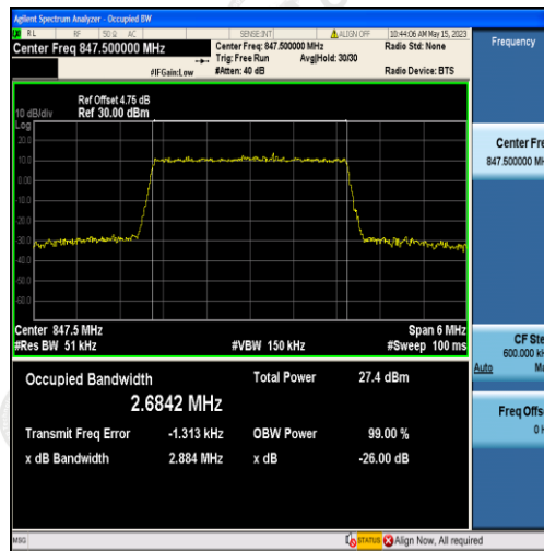
Band5-3MHz-QPSK-20635-15RB#0-2.6842
