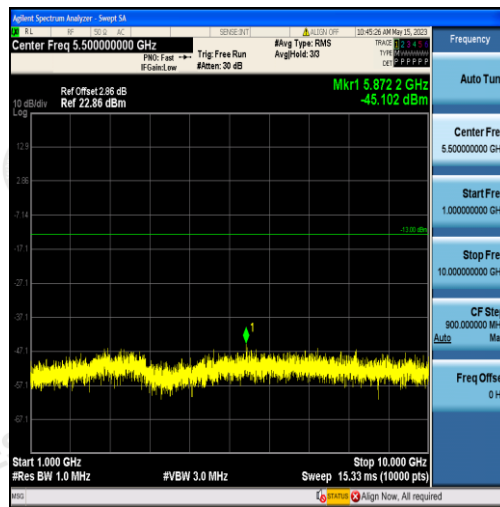
Band5-3MHz-QPSK-20415-15RB#0-Range2:1000~10000MHz
