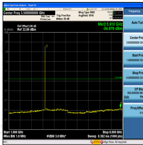
Band38-5MHz-QPSK-38000-25RB#0-Range2:1000~6000MHz
