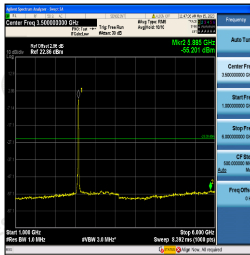
Band38-20MHz-QPSK-37850-100RB#0-Range2:1000~6000MHz
