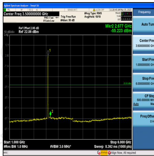
Band38-10MHz-QPSK-37800-50RB#0-Range2:1000~6000MHz
