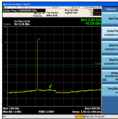
Band38-10MHz-QPSK-38200-50RB#0-Range2:1000~6000MHz
