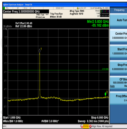
Band38-20MHz-16QAM-37850-100RB#0-Range2:1000~6000MHz
