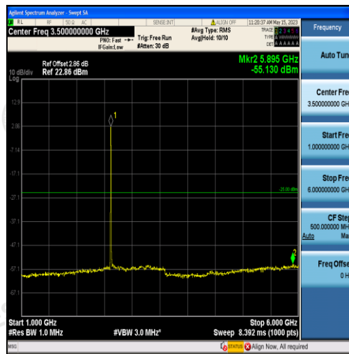
Band38-5MHz-QPSK-38225-25RB#0-Range2:1000~6000MHz
