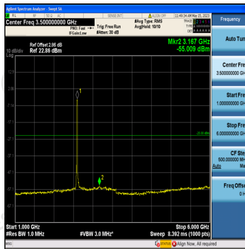
Band38-20MHz-QPSK-38000-100RB#0-Range2:1000~6000MHz
