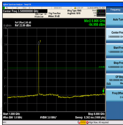
Band38-10MHz-QPSK-38000-50RB#0-Range2:1000~6000MHz
