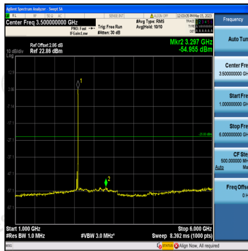
Band41-5MHz-QPSK-40620-25RB#0-Range2:1000~6000MHz
