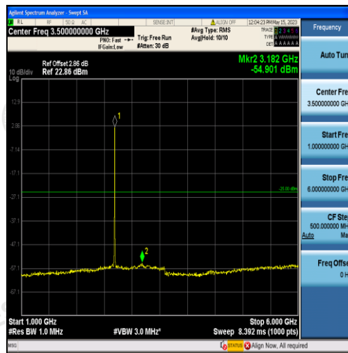
Band41-5MHz-QPSK-41565-25RB#0-Range2:1000~6000MHz
