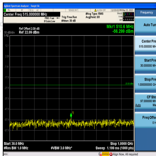
Band41-5MHz-QPSK-40620-25RB#0-Range1:30~1000MHz
