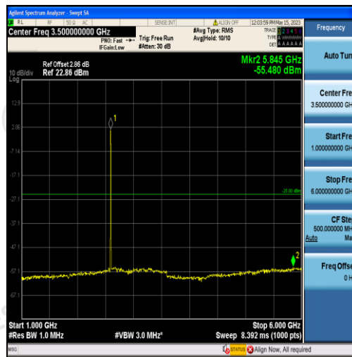
Band41-5MHz-16QAM-40620-25RB#0-Range2:1000~6000MHz
