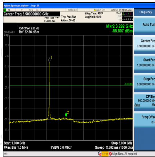
Band38-20MHz-QPSK-38150-100RB#0-Range2:1000~6000MHz
