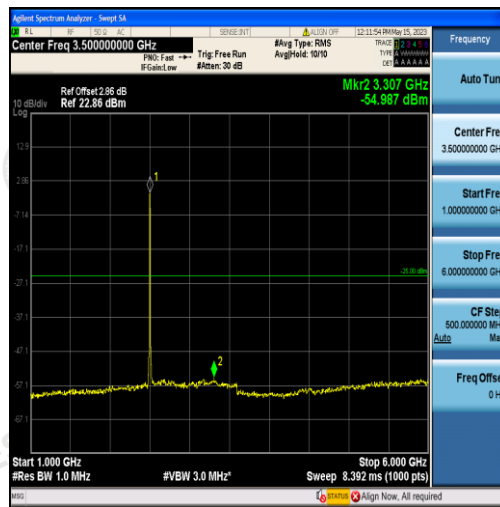
Band41-10MHz-QPSK-39700-50RB#0-Range2:1000~6000MHz
