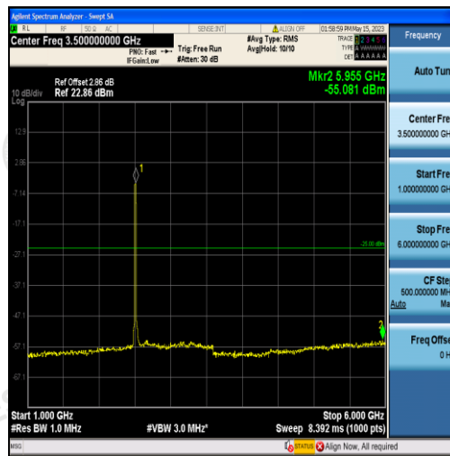
Band41-20MHz-QPSK-39750-100RB#0-Range2:1000~6000MHz
