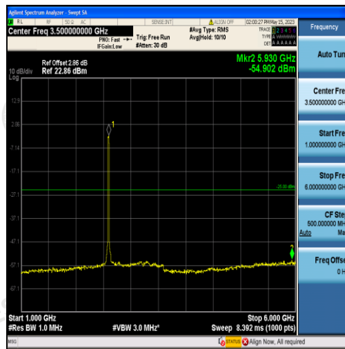
Band41-20MHz-QPSK-40620-100RB#0-Range2:1000~6000MHz
