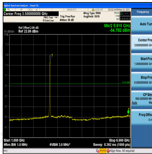
Band41-20MHz-QPSK-41490-100RB#0-Range2:1000~6000MHz
