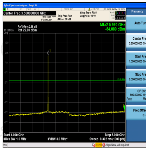
Band41-10MHz-16QAM-41540-50RB#0-Range2:1000~6000MHz
