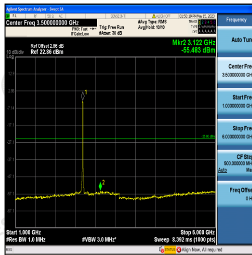
Band41-15MHz-QPSK-41515-75RB#0-Range2:1000~6000MHz
