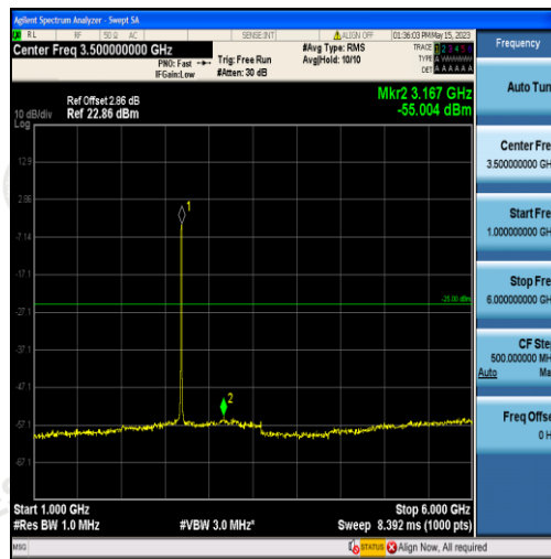
Band41-10MHz-QPSK-41540-50RB#0-Range2:1000~6000MHz
