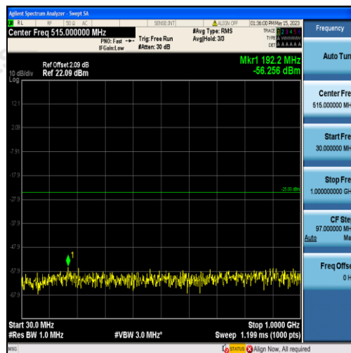
Band41-10MHz-QPSK-41540-50RB#0-Range1:30~1000MHz
