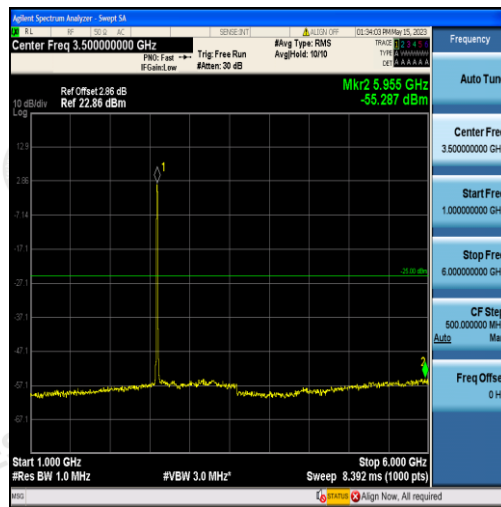
Band41-10MHz-QPSK-40620-50RB#0-Range2:1000~6000MHz
