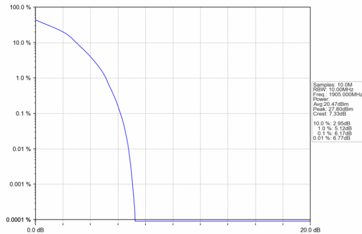
Band2 10MHz 16QAM HCH 1905MHz RB 27 23 NTNV
