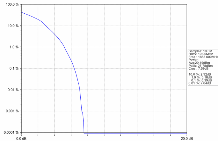
Band2 10MHz 16QAM LCH 1855MHz RB 27 0 NTN
