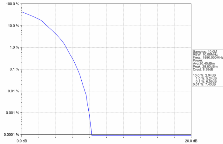
Band2 10MHz 16QAM MCH 1880MHz RB 27 0 NTNV
