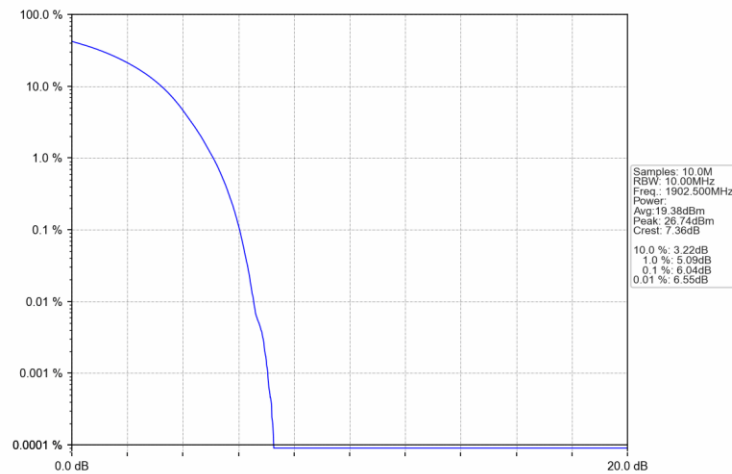
Band2 15MHz 16QAM HCH 1902.5MHz RB 27 48 NTNV
