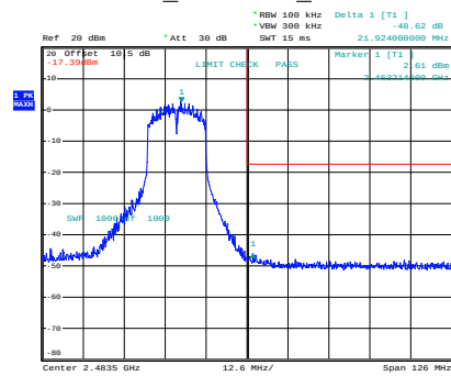
n20_2462MHz_Chain 0
