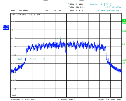
n20_2462MHz_Chain 0
