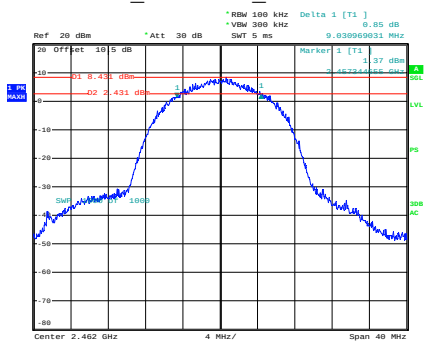
b_2462MHz_Chain 0
