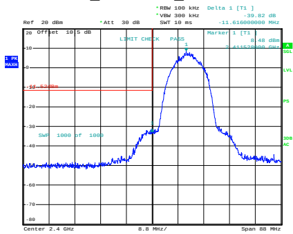
b_2412MHz_Chain 0
