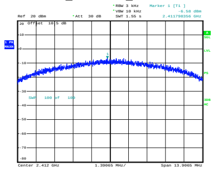
b_2412MHz_Chain 0
