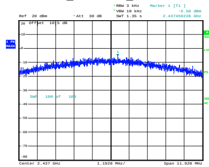
b_2437MHz_Chain 0
