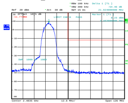
b_2462MHz_Chain 0
