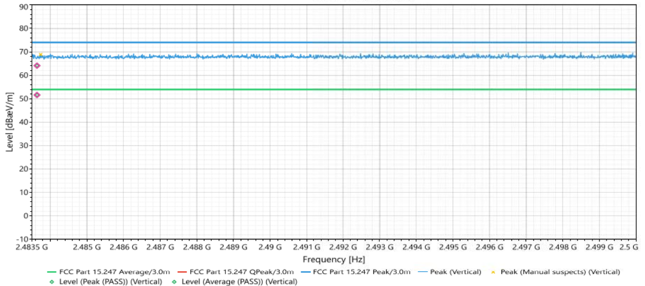
#1 - 2.4835GHz-2.5GHz (Vertical)
