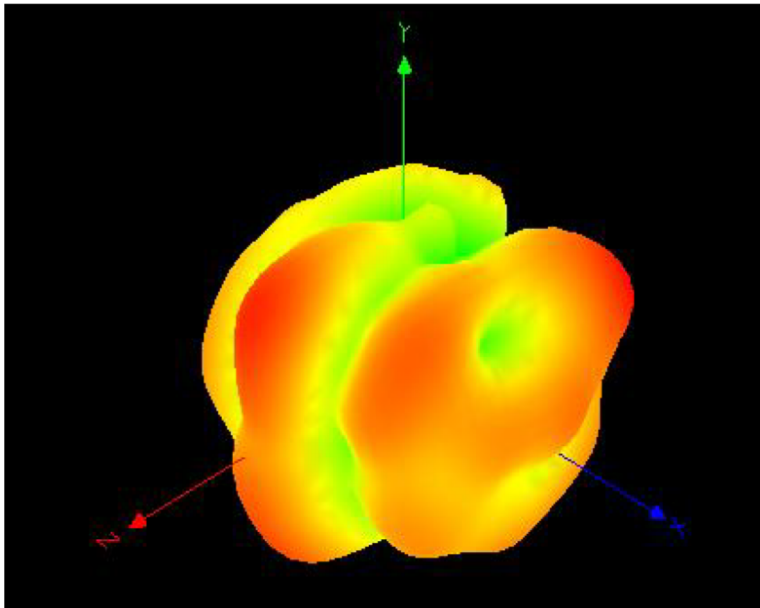
PCS 1900& WCDMA Band 2& LTE Band 2
