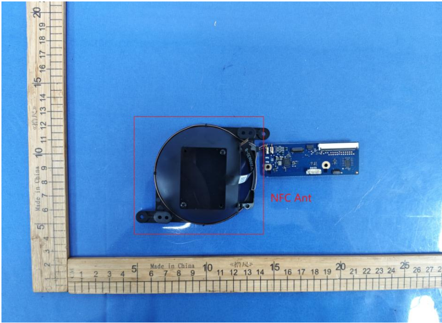
NFC Antenna
