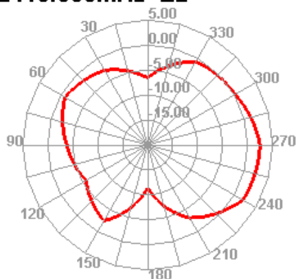
2410.000MHz E2
