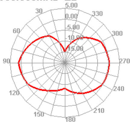
900.000MHz E2
