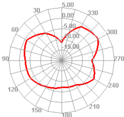
2680.000MHz H
