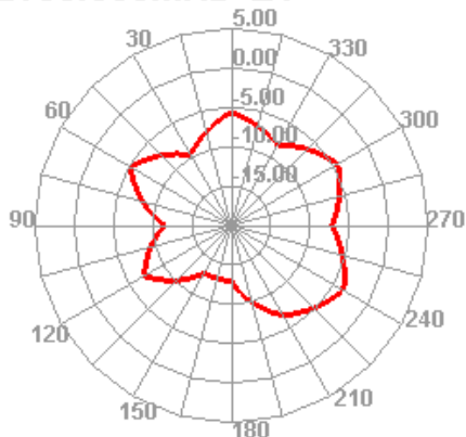
2680.000MHz E1
