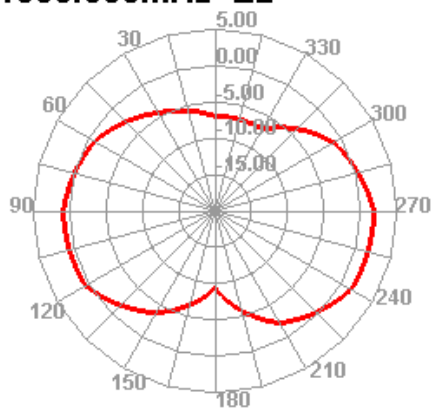
1800.000MHz E2
