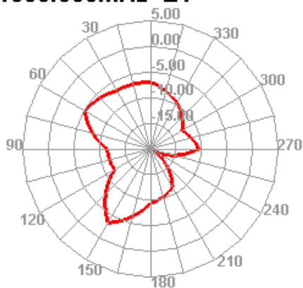
1800.000MHz E1
