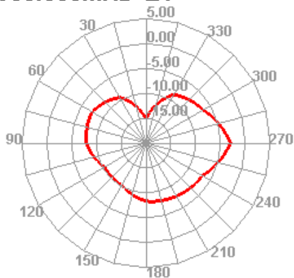
900.000MHz E1
