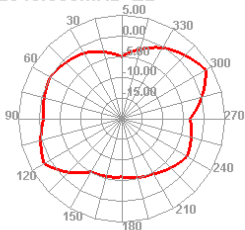
2540.000MHz E2
