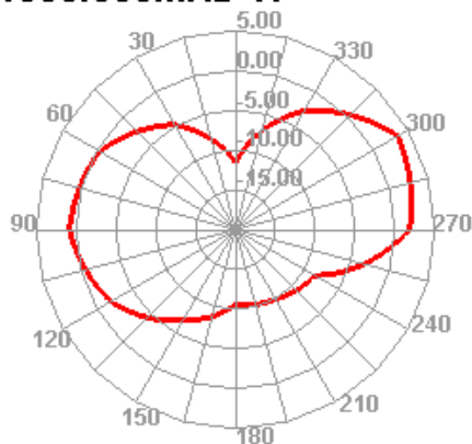
1800.000MHz H
