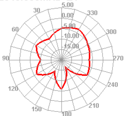
2540.000MHz E1
