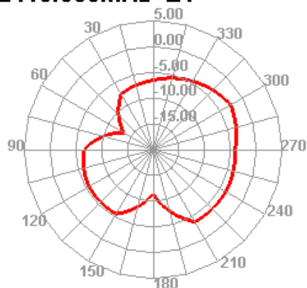
2410.000MHz E1
