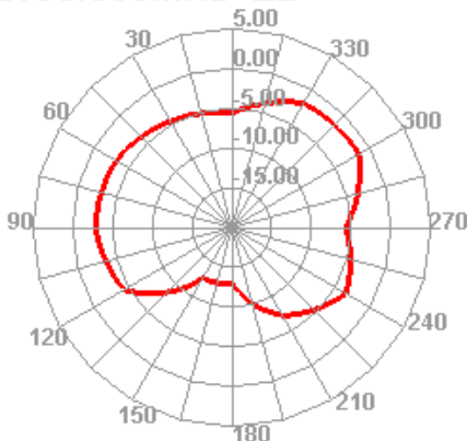
2680.000MHz E2
