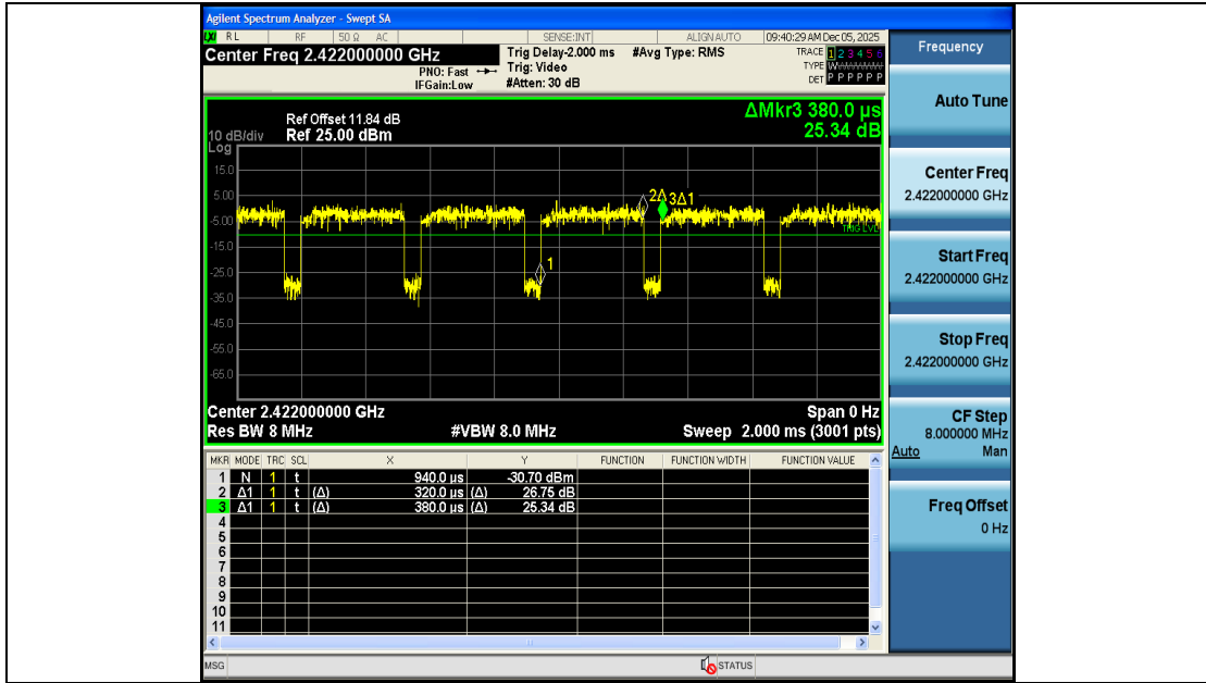
NTNV-11N40-Ant2-2422
