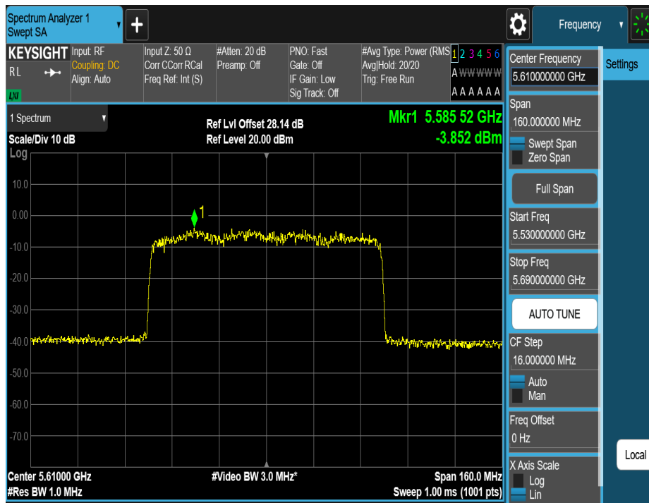
11AX80MIMO_Ant2_5610
