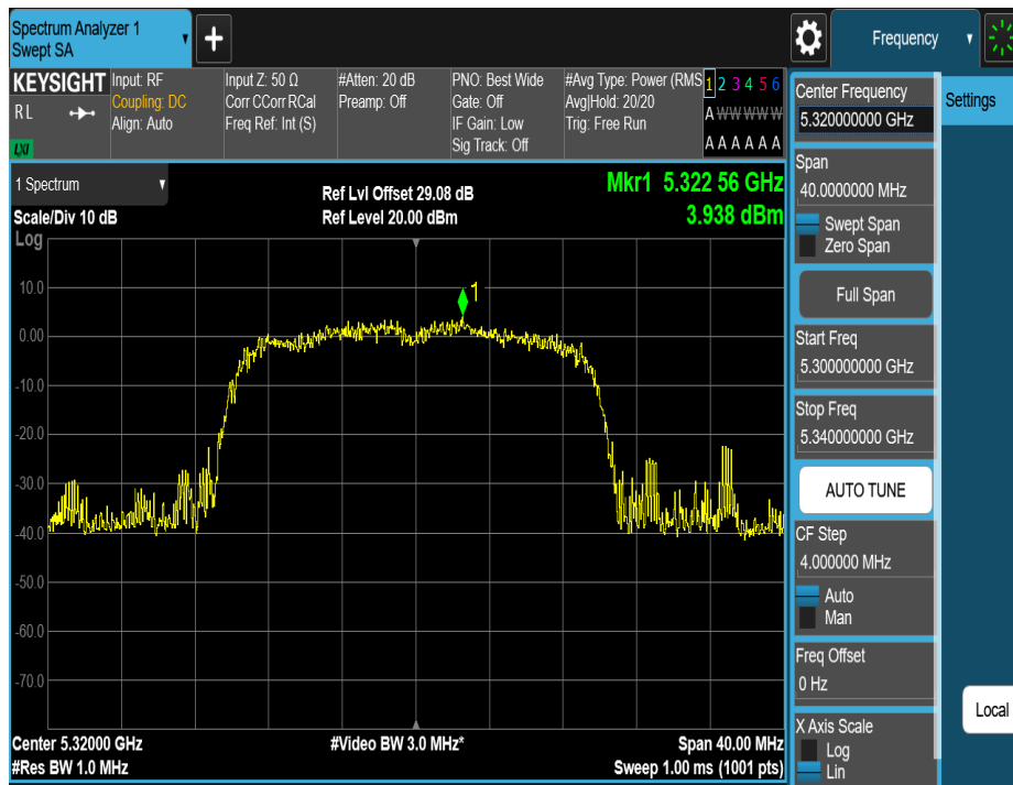
11AX20MIMO_Ant2_5320
