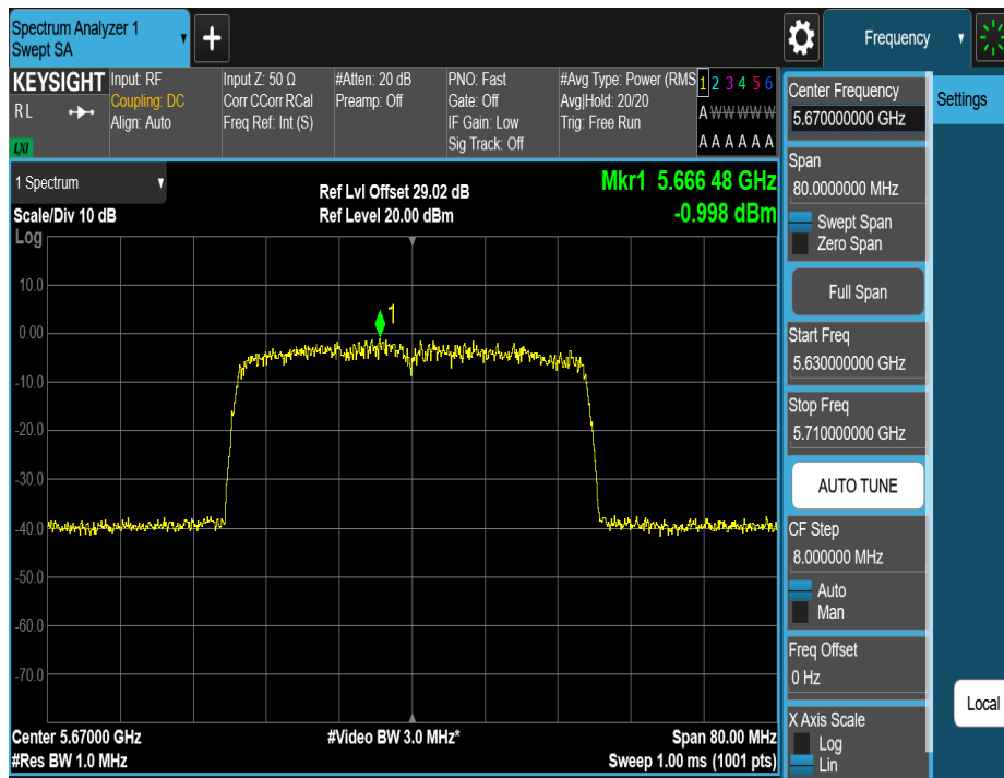
11AX40MIMO_Ant2_5670
