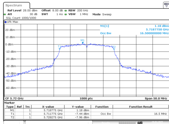
802.11a_5720MHz_Chain 0
