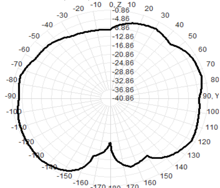
2500.0MHz Total(E2-YZ), Max=-1.23dB
