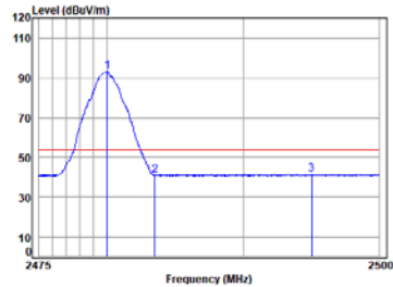
BLE_2M_TX_CH_39_Horizontal-Avg
