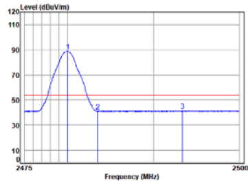
BLE_2M_TX_CH_39_Vertical-Avg
