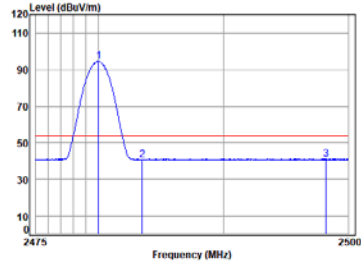
BLE_1M_TX_CH_39_Horizontal-Avg
