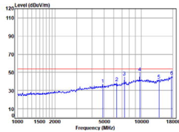
BLE_2M_TX_CH_19_Vertical-Avg
