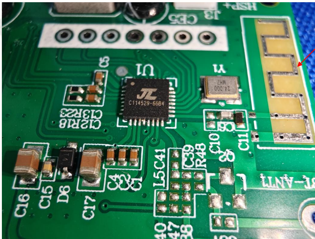
BT: PCB Antenna
