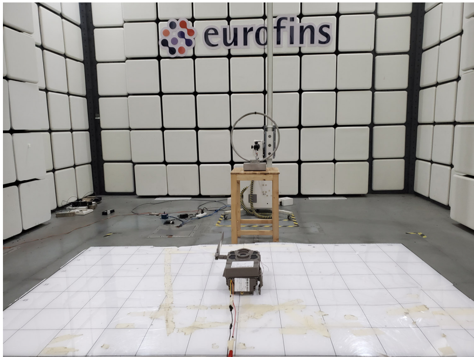
9kHz-30MHz
