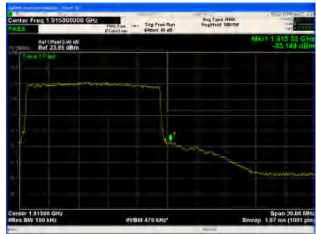
LTE Band 25 20MHz QPSK 1RB CH-High
