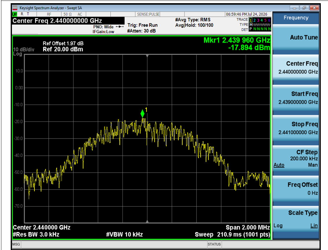
PSD NVNT BLE 1M 2440MHz Ant1
